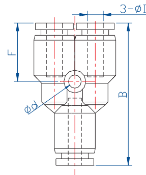
Y Union, YU
